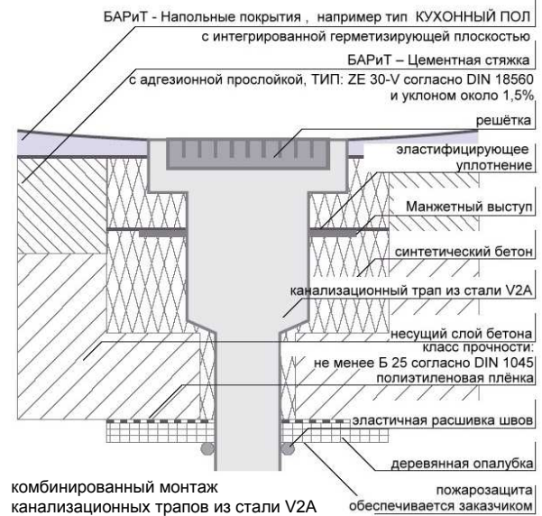
монтаж канализационных трапов из стали V2A на уровне грунта
