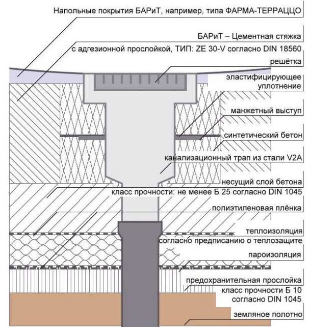
монтаж канализационных трапов из стали V2A на уровне грунта
