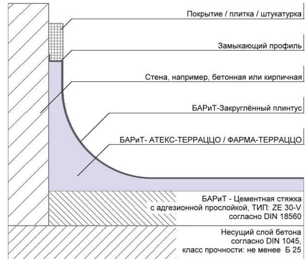
Плинтус как элемент комбинированной конструкции Плинтус в сочетании с напольным покрытием Пауэр
