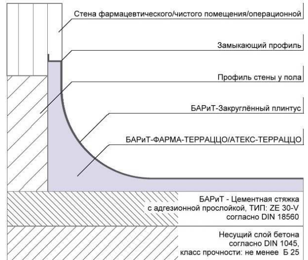
Плинтус как элемент комбинированной конструкции
