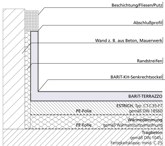
Senkrechtsockel mit Randstreifen
