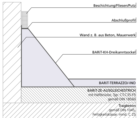
Dreikantsockel im Verbund
