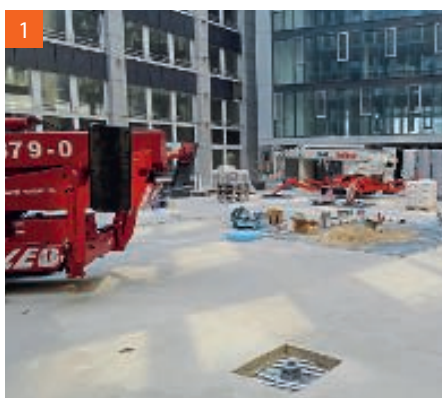
1 Damit die Fassadenflächen im inneren Bereich ausgeführt werden konnten, waren zeitweise drei Arbeitsbühnen im Einsatz. Aussparungsbereiche wurden nachträglich mit einem hochwertigen Epoxidharzestrichmörtel verfüllt.
